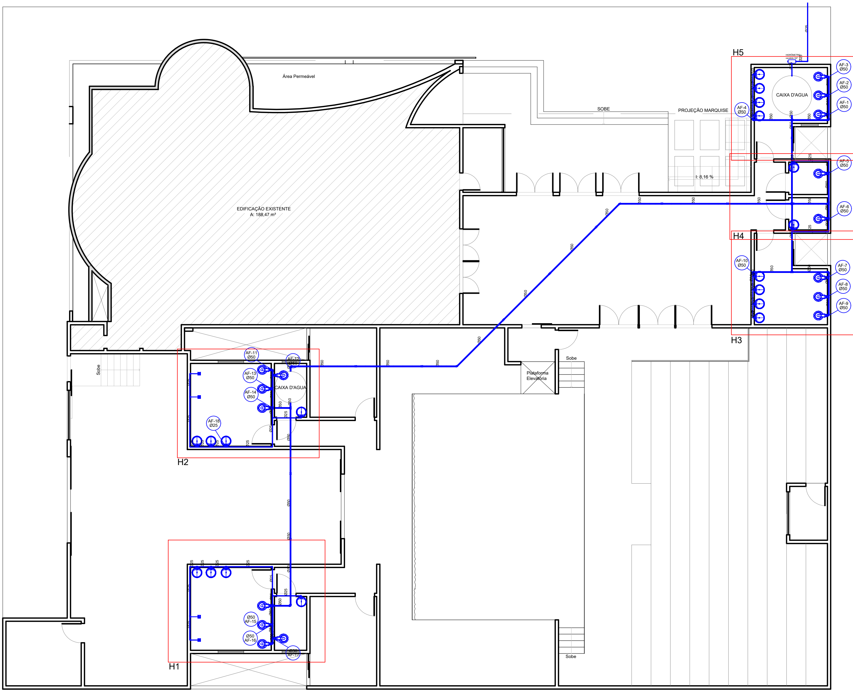
PLANTA HIDRÁULICA ESC.: 1/100
