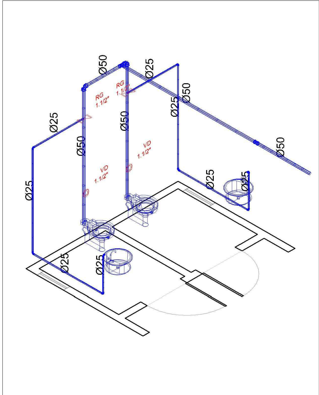
DETALHE H4 s/ escala
