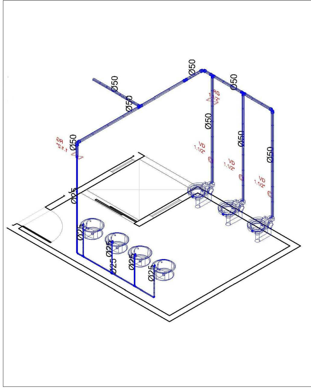
DETALHE H3 s/ escala
