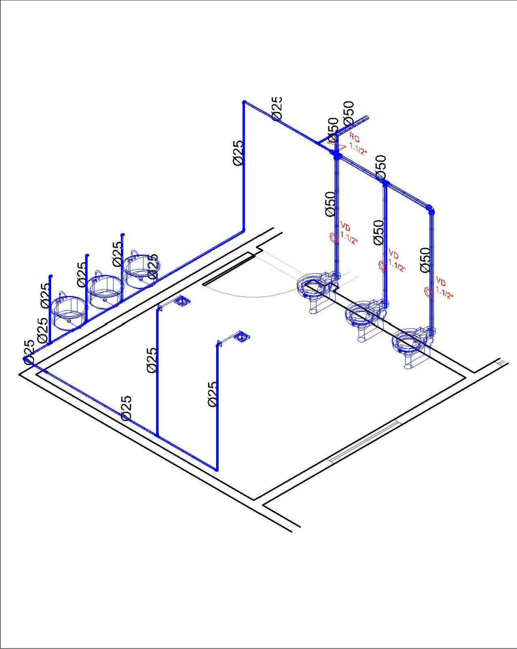
DETALHE H1 s/ escala
