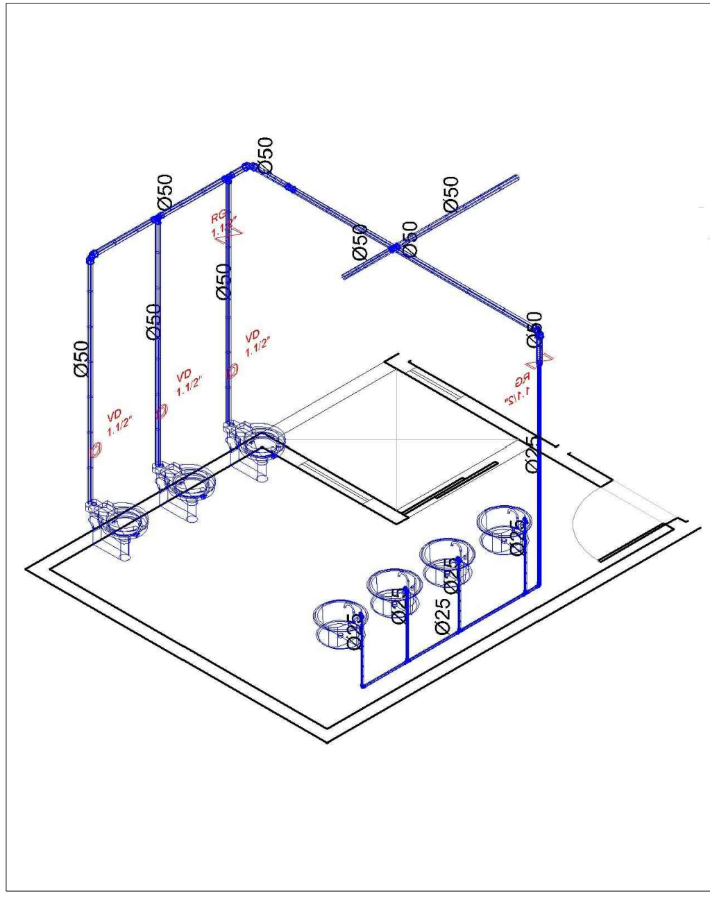
DETALHE H5 s/ escala
