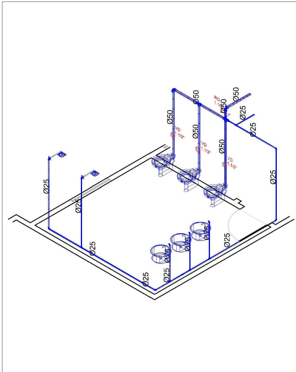
DETALHE H2 s/ escala
